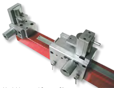
Vorrichtung zur Längenprüfung von Gerüstbauteilen.
