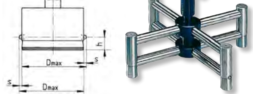
Kreuzkufenhülse auf Anfrage. Cross sleeve on request.
